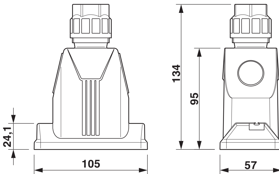
Disegno quotato
