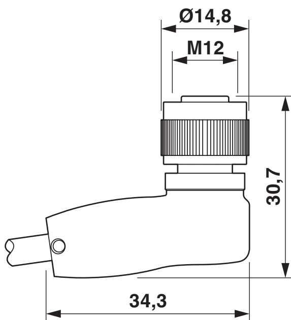
Disegno quotato
