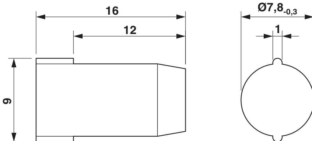
Disegno quotato
