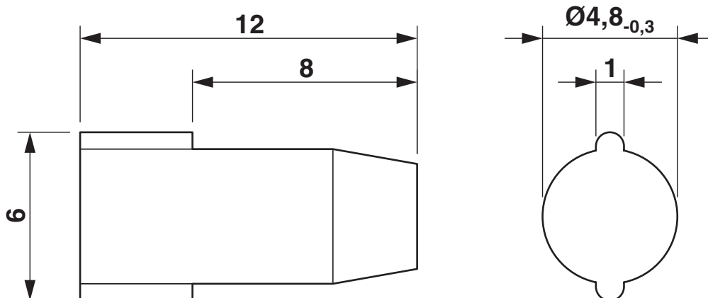
Disegno quotato
