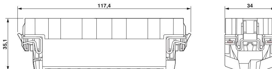
Disegno quotato
