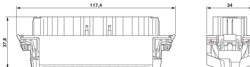
Disegno quotato
