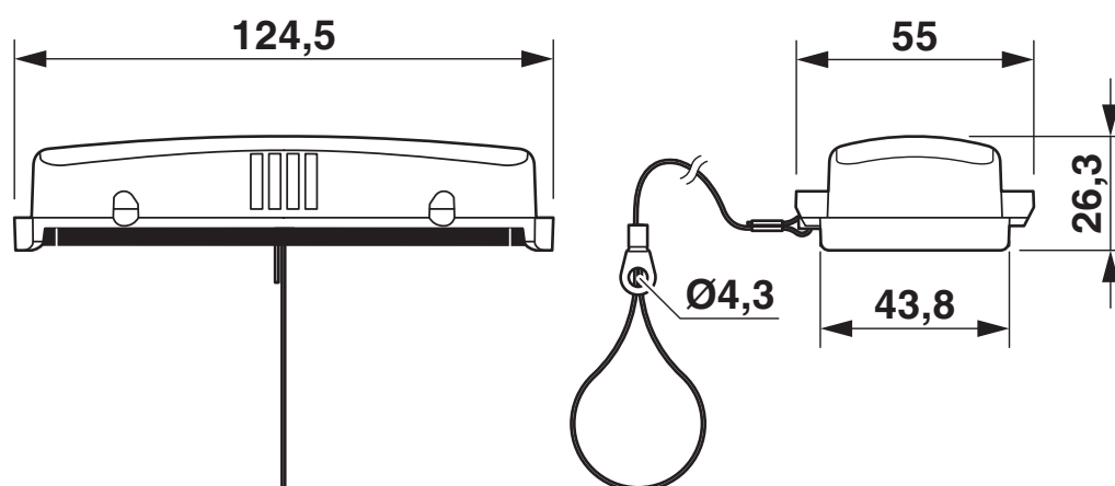
Disegno quotato
