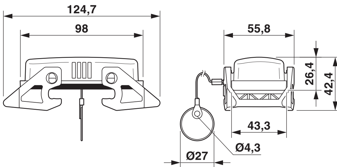
Disegno quotato
