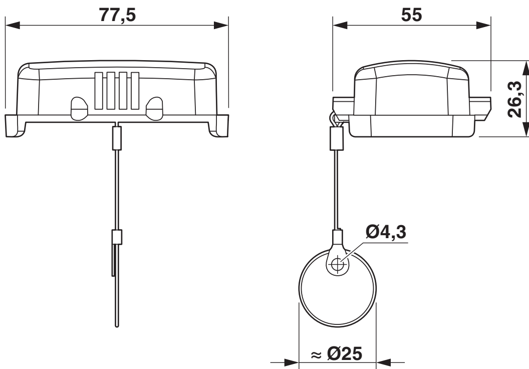
Disegno quotato
