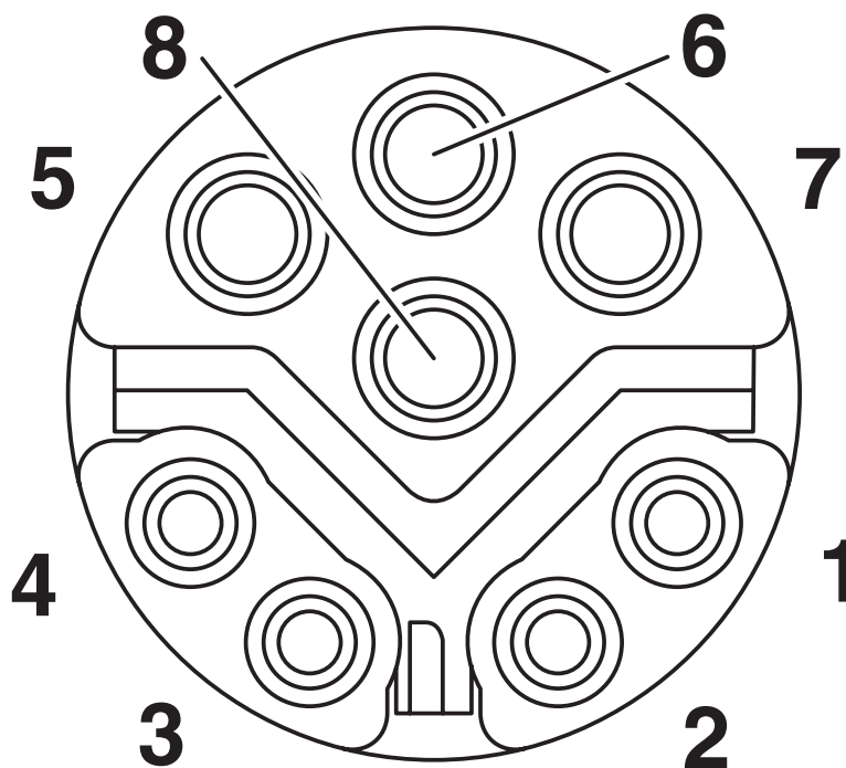
Disegno schema
