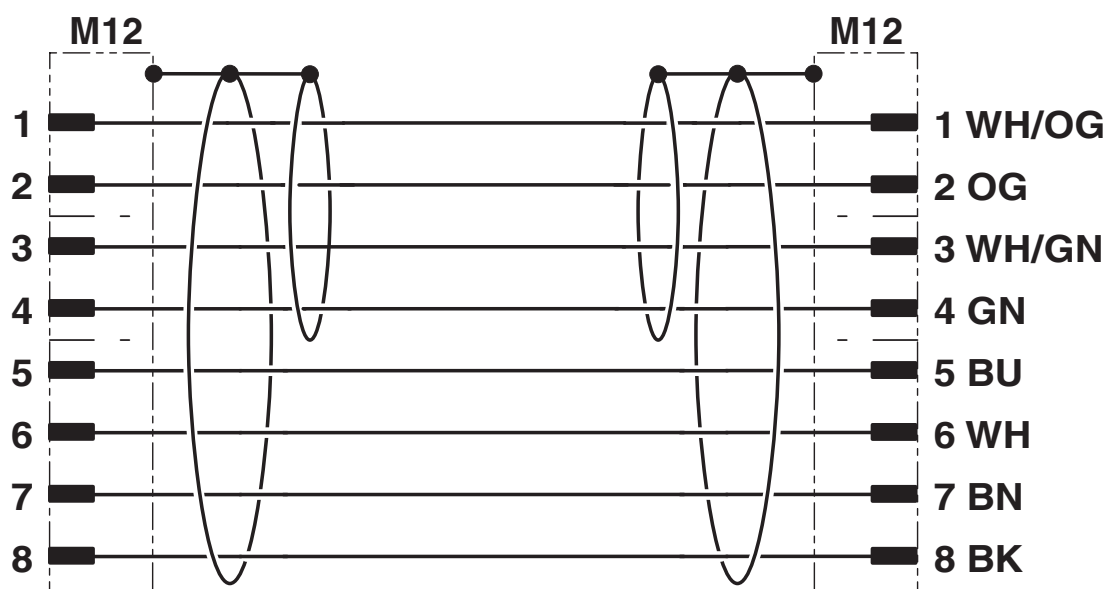
Equipaggiamento dei contatti del connettore M12
