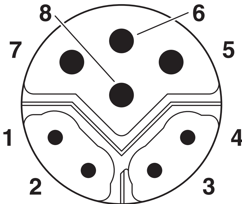
Disegno schema
