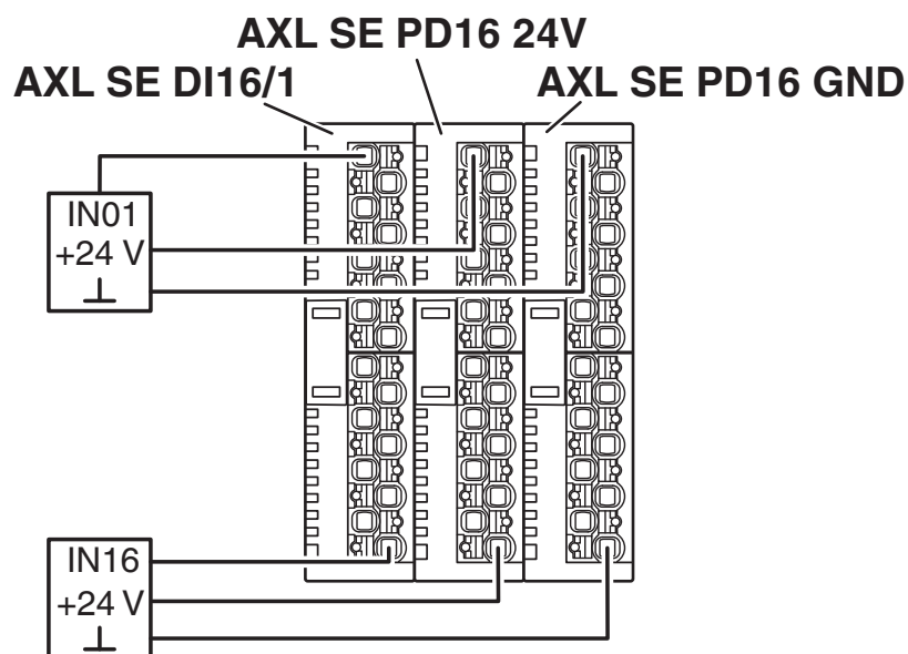
Disegno collegamento
