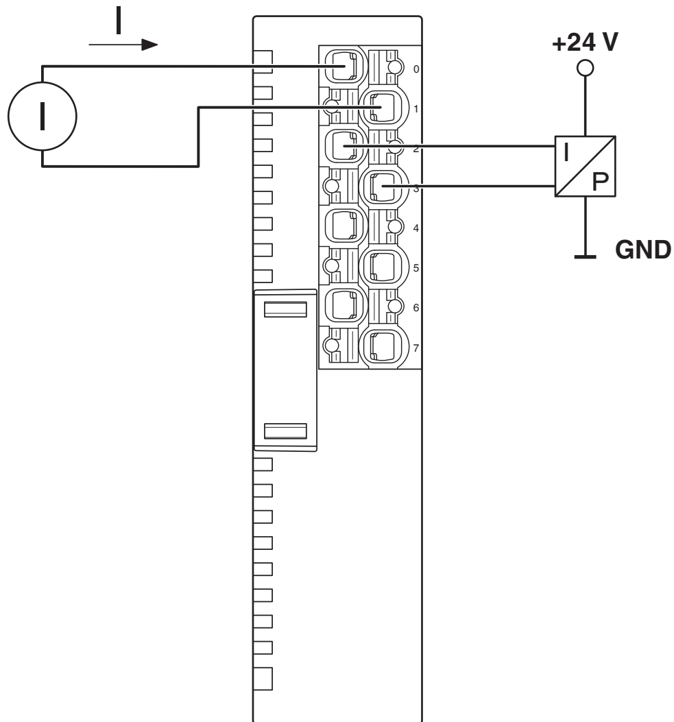
Disegno collegamento
