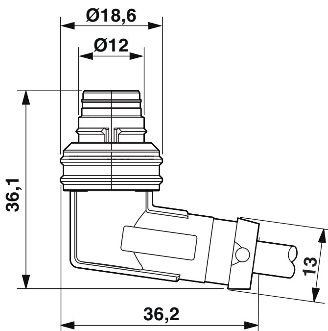
Connettore maschio Push-Pull M12, angolato, schermato
