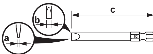
Disegno quotato
