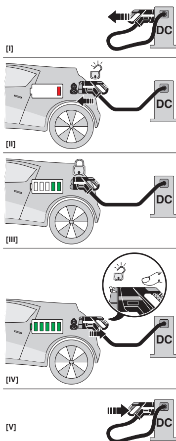
Disegno schema
