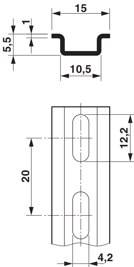
Disegno quotato
