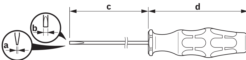
Disegno quotato
