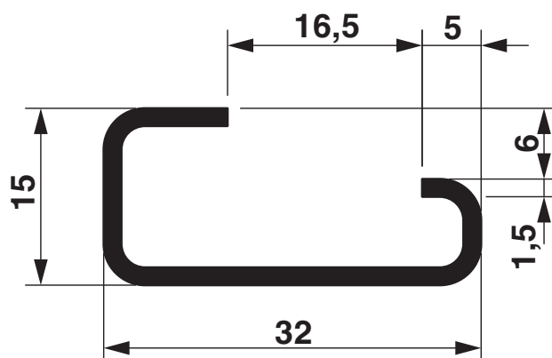
Disegno quotato
