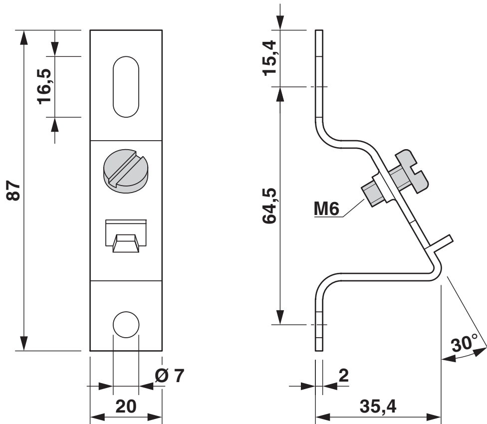
Disegno quotato
