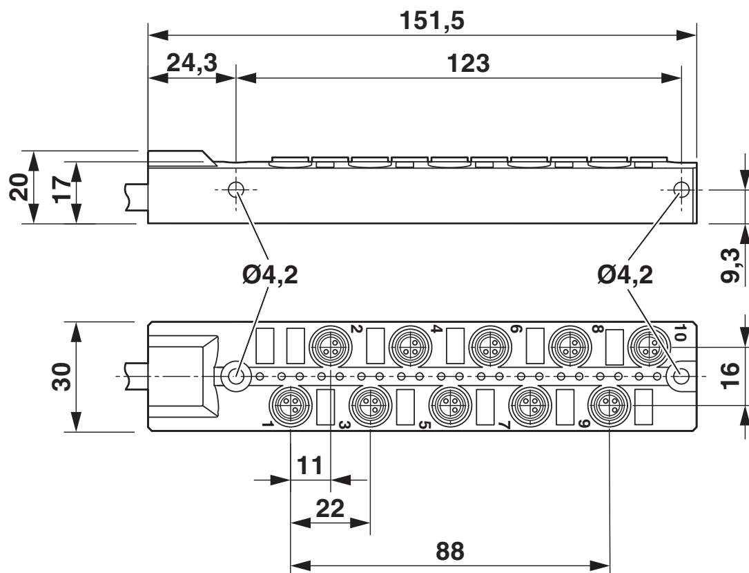
Disegno quotato
