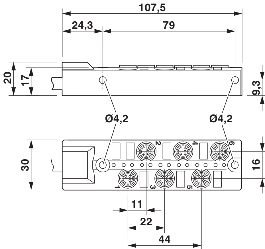
Disegno quotato
