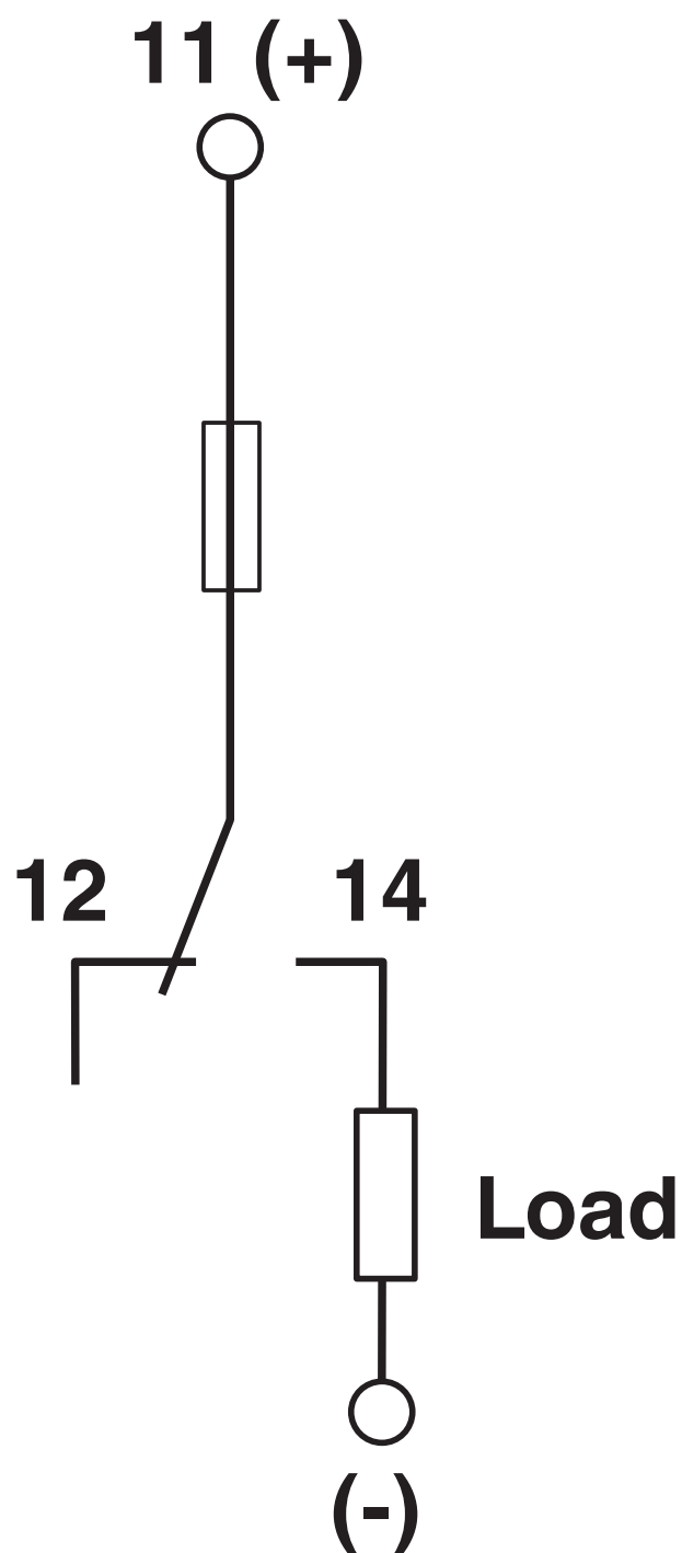
Schema di collegamento
