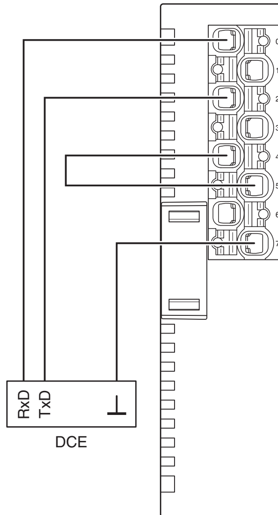
Disegno collegamento
