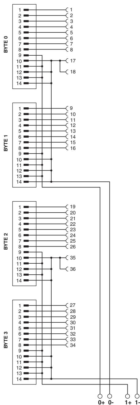
Schema di collegamento
