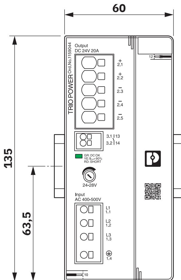
Disegno quotato
