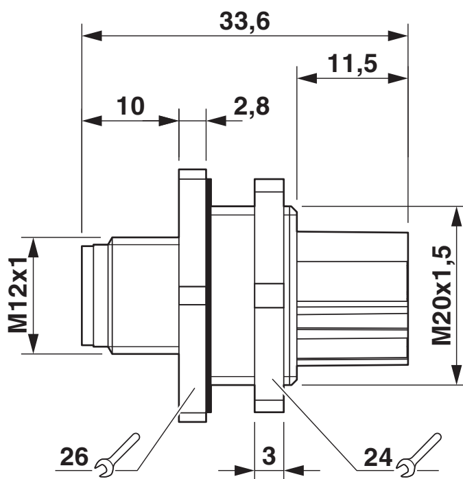
Disegno quotato
