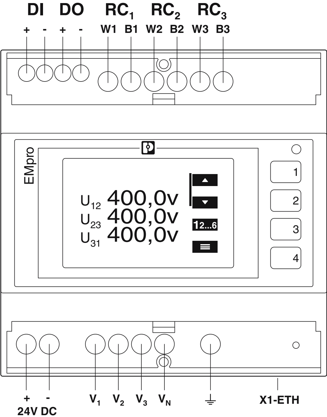
Disegno collegamento
