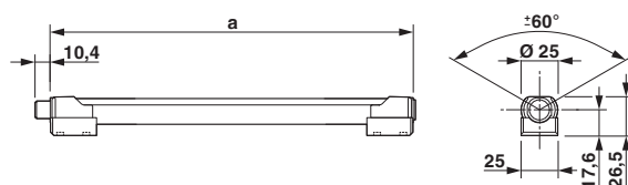
Disegno quotato
