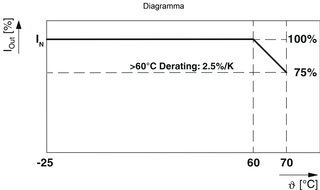
Corrente d'uscita/temperatura ambiente
