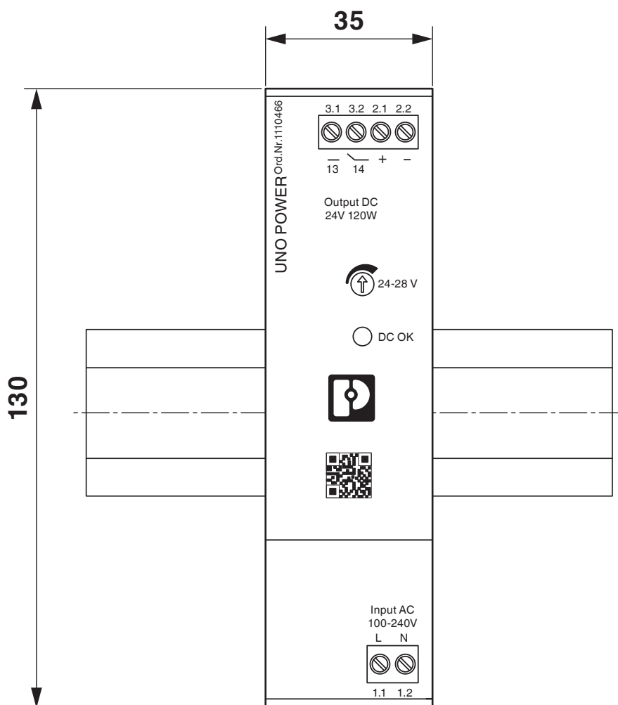
Disegno quotato
