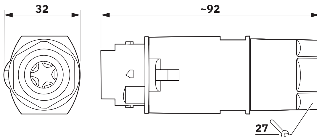
Disegno quotato
