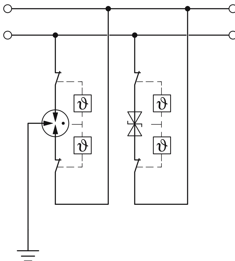
Disegno collegamento
