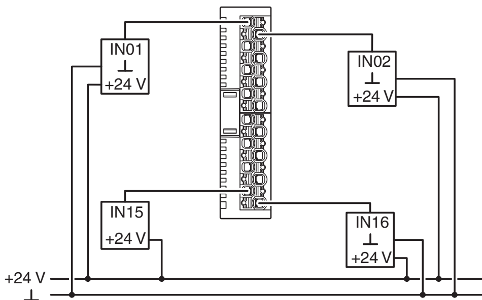
Disegno collegamento
