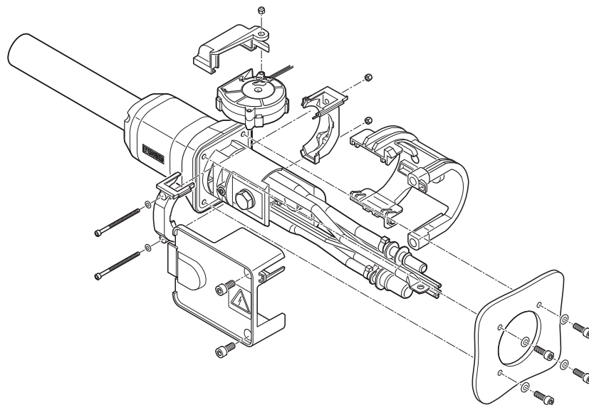
Disegno schema
