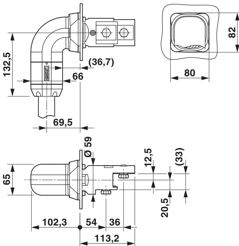
Disegno quotato
