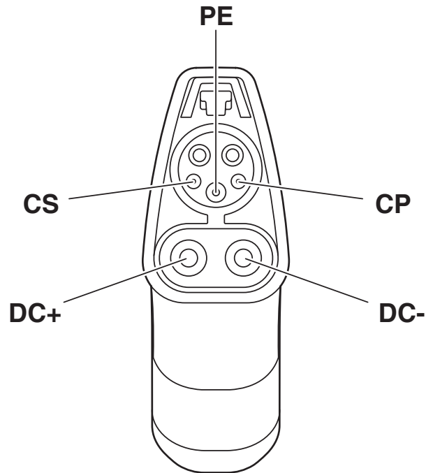
Disegno schema
