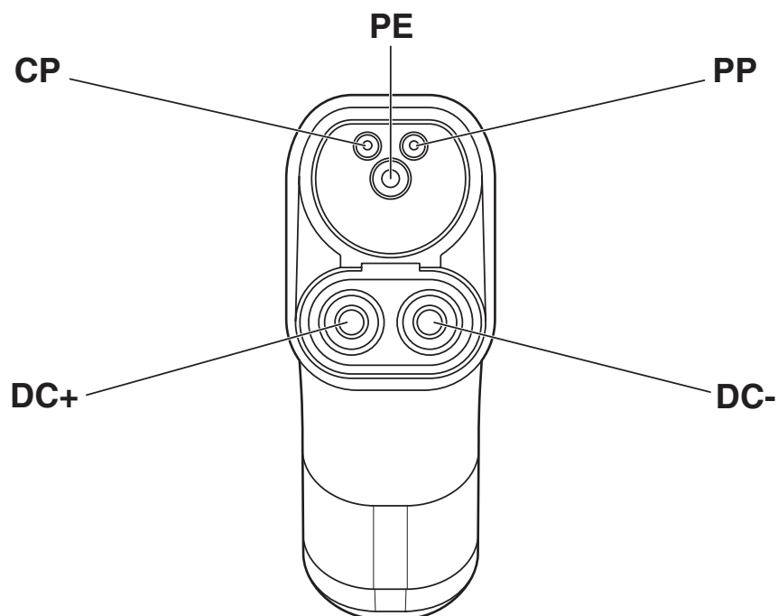
Piedinatura connettore di ricarica infrastruttura
