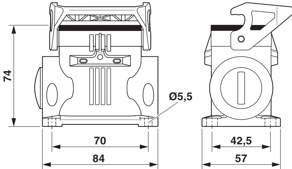
Disegno quotato
