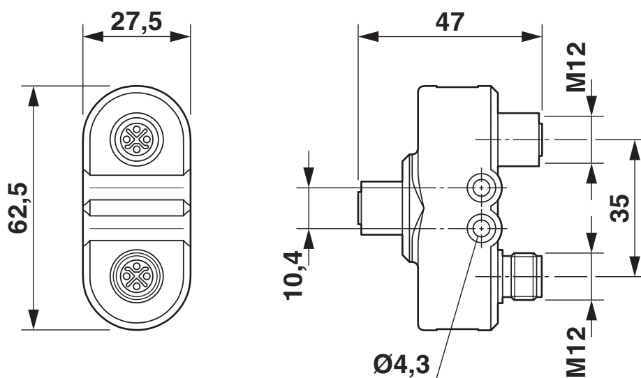
Disegno quotato
