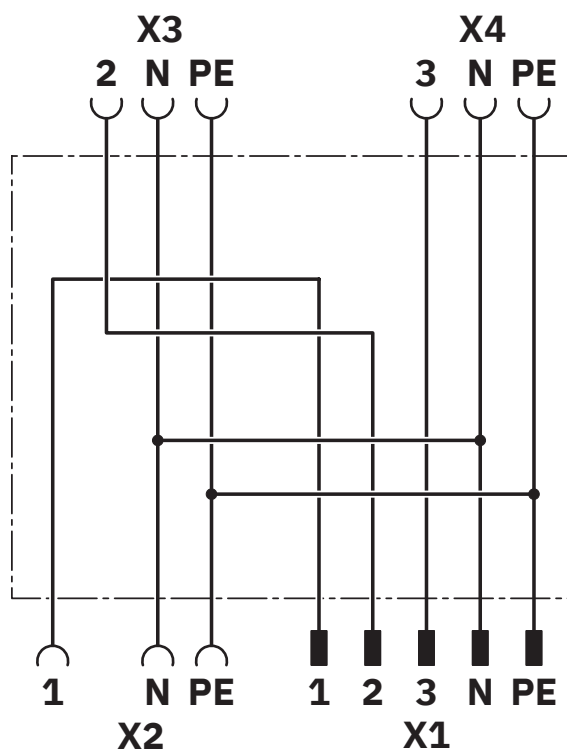
Schema di collegamento
