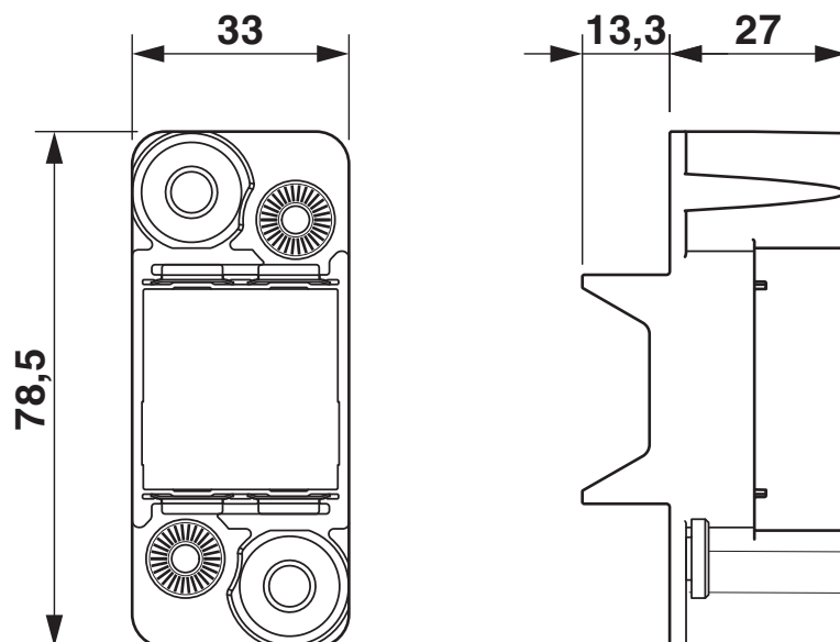
Disegno quotato
