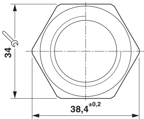
Disegno quotato
