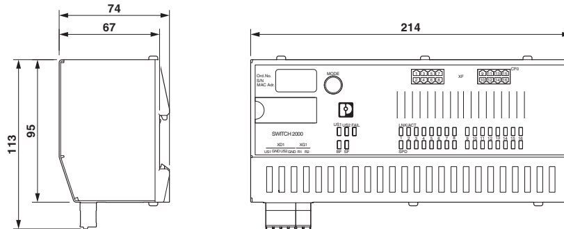
Disegno quotato
