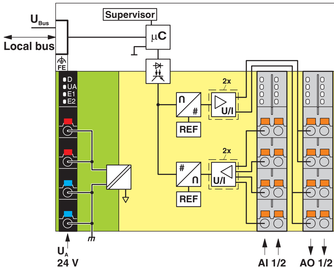
Circuito interno dei punti di connessione
