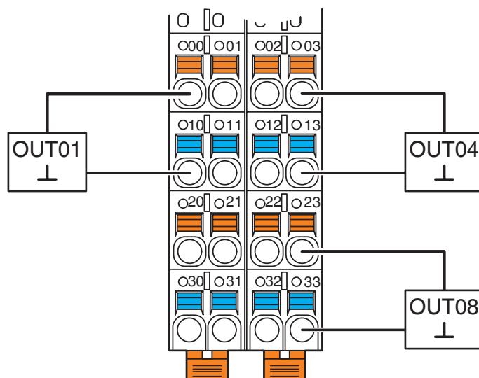
Disegno collegamento
