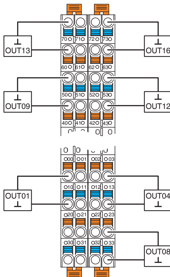
Disegno collegamento
