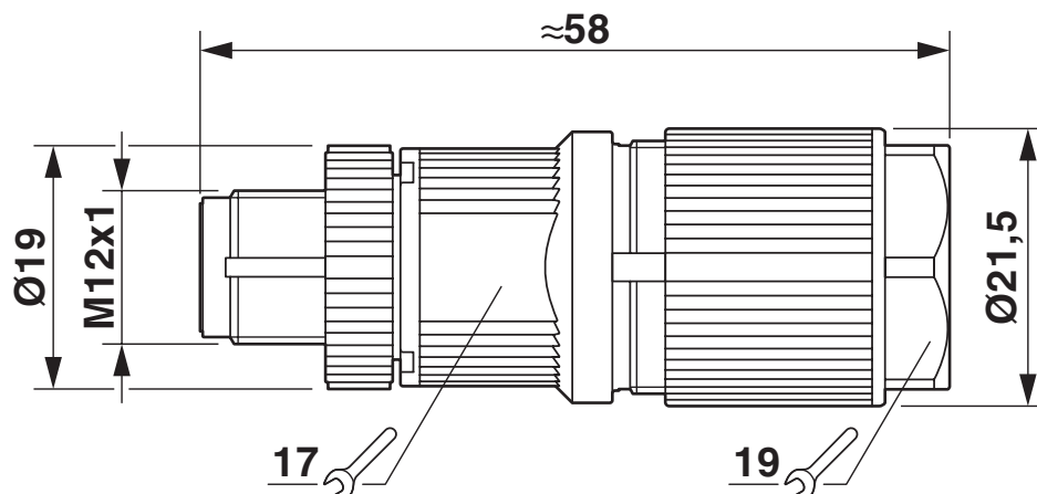
Disegno quotato
