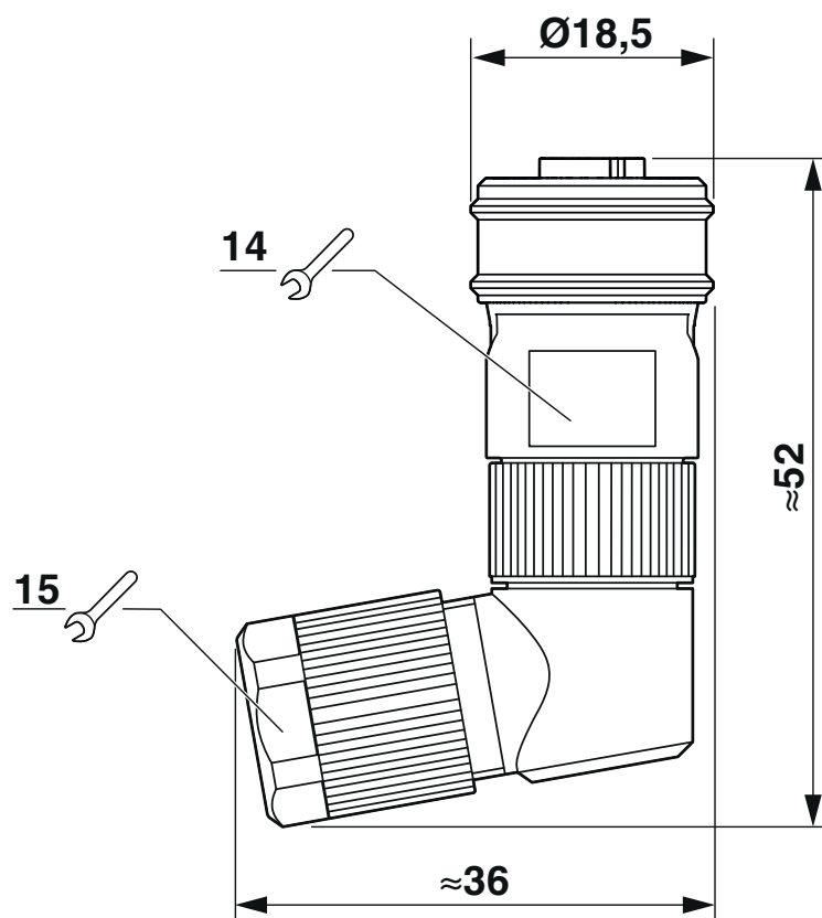
Connettore femmina M12 Push-Pull, angolato, schermato
