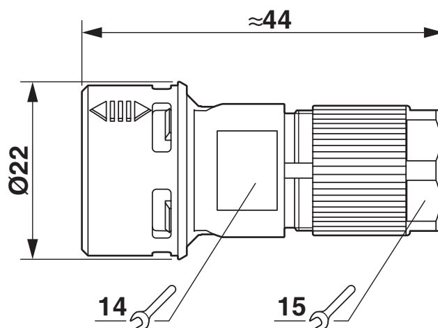
Disegno quotato
