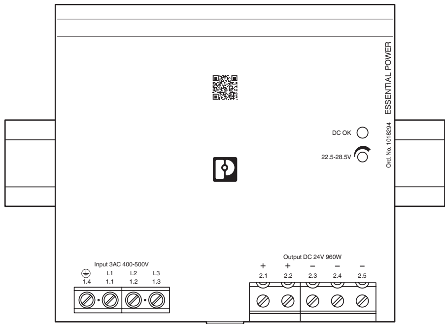
Disegno schema
