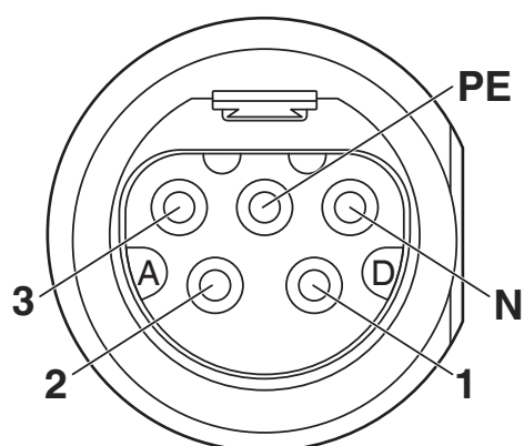
Disegno schema
